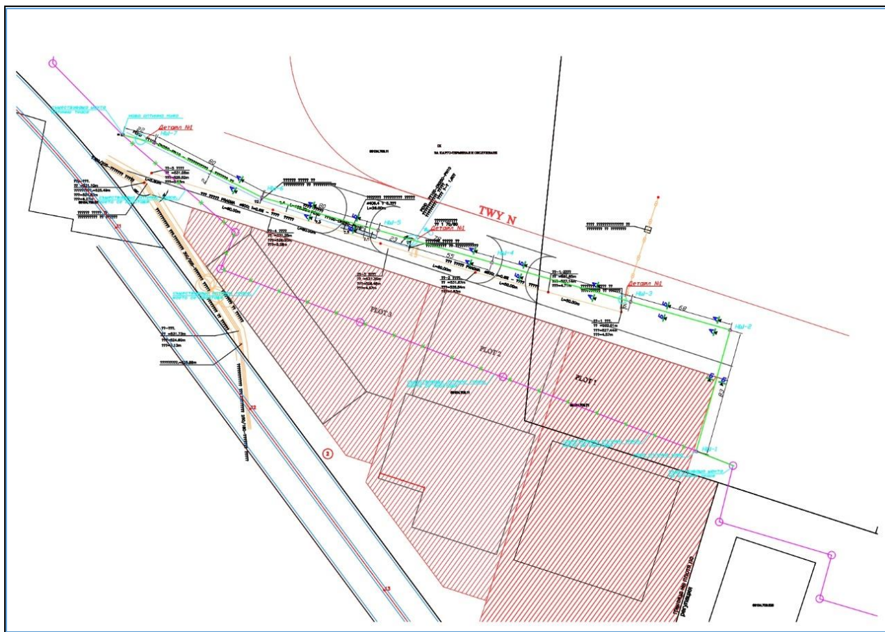
Фигура 2. Съществуващо и изместено трасе на оптичен кабел (маркировка в мангента за съществуващо трасе и маркировка в зелено за ново трасе)
