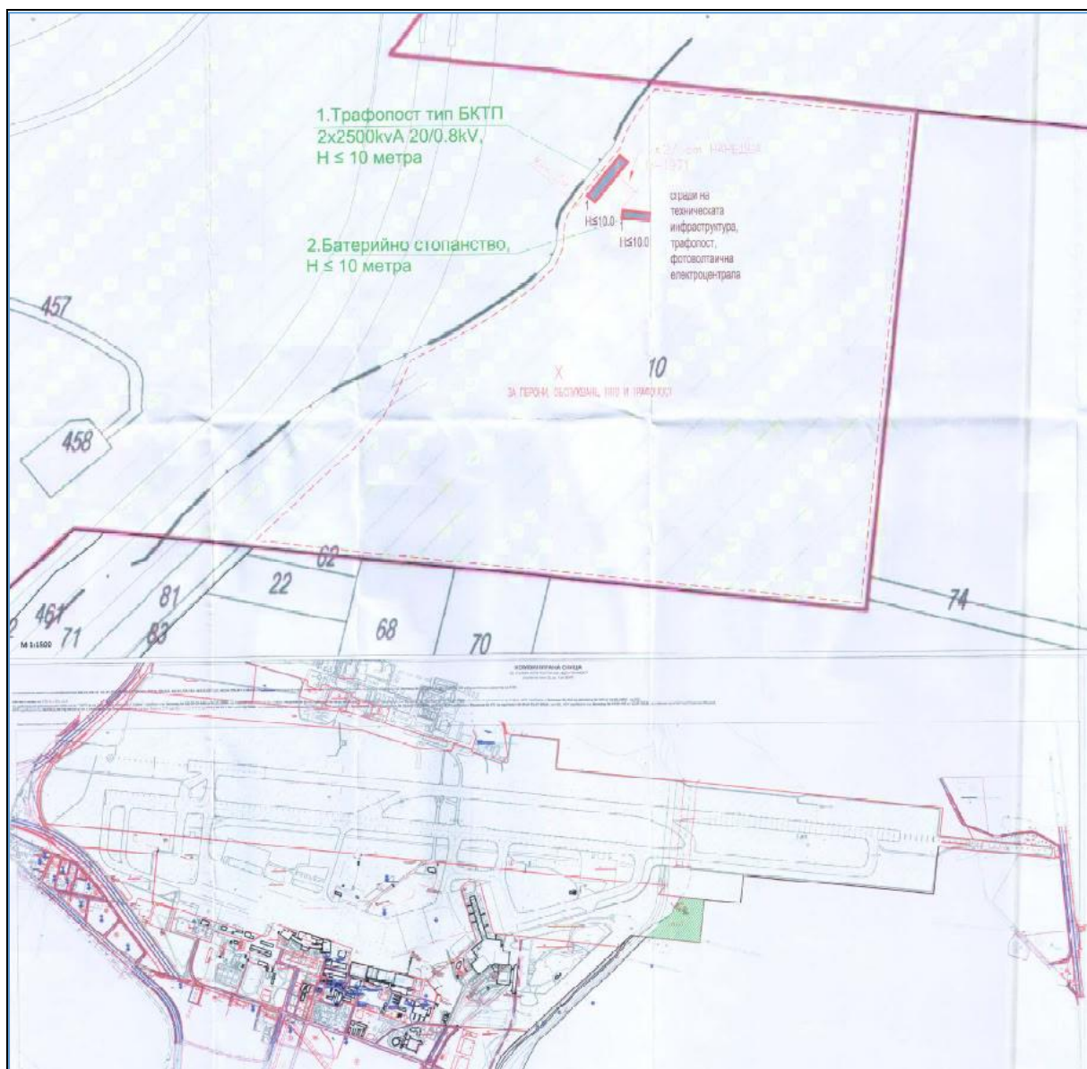
Фигура 9. Разположение на батерийното стопанство
