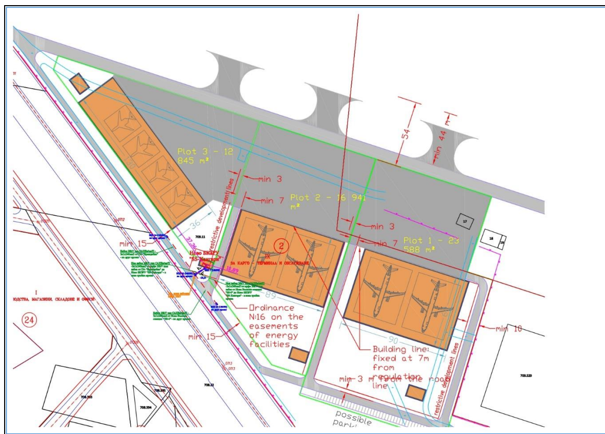
Фигура 5. Местоположение нова БКЗРУ "SS-Хангари"
