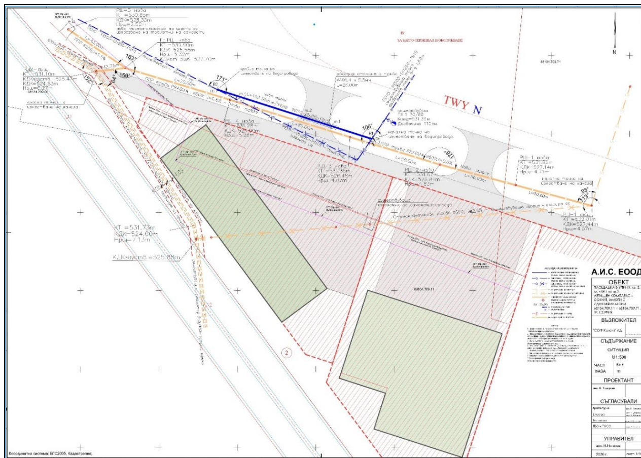
Фигура 4. Ново трасе за изместване на съществуващ канализационен клон (маркировка в кафяво)
