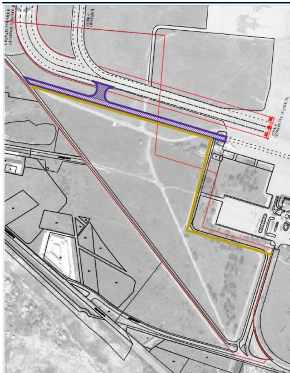
Фигура 6. Нова ограда за изместване на границата между страна „Земля“ и страна „Въздух“ (маркировка в жълто)
