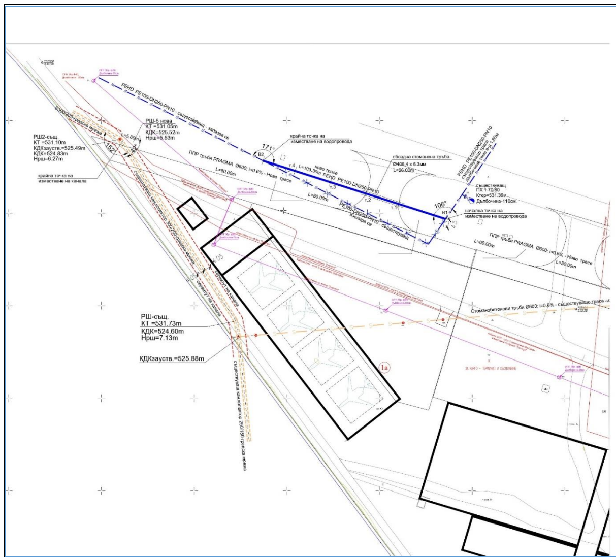
Фигура 3. Изместване на вътрешно-площадков водопровод (маркировка в синьо)
